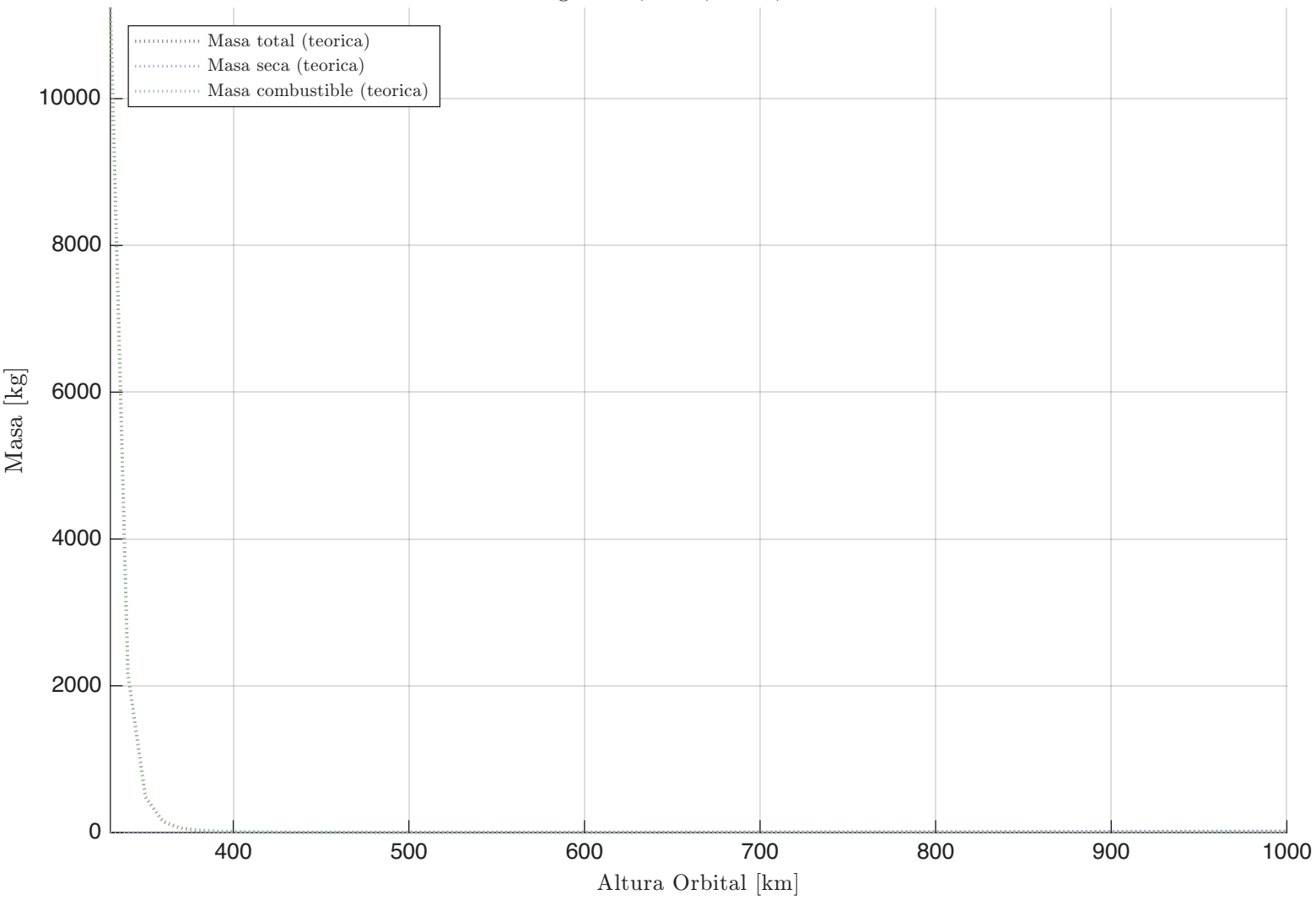
Desglose de Masas vs. Altura Config: 1 Sat, 1 Tel, Det 1, Refractivo
